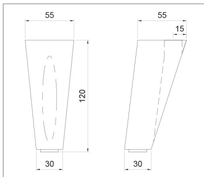
739R műanyag bútorláb M8-as furattal
