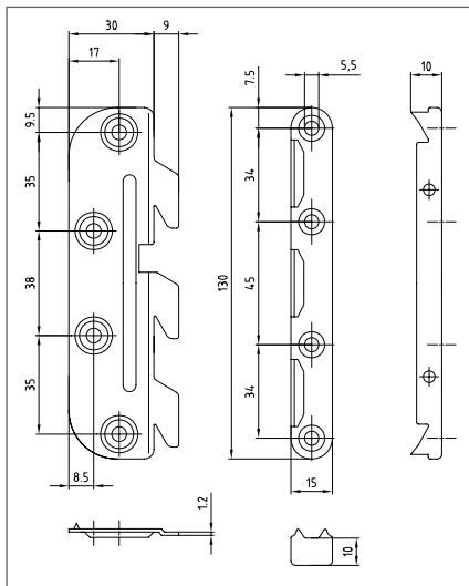
3361.0000.30 ágyvasalat
