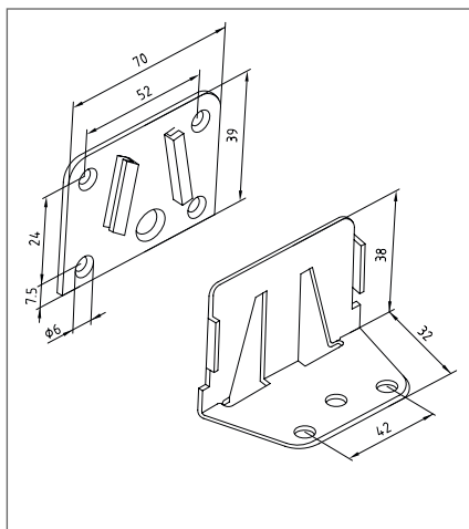
3892.0000.30 ágyvasalat
