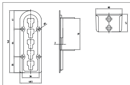
3366.0000.30 ágyvasalat
